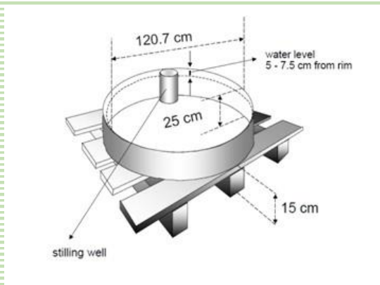
شکل ۹- نمایی از یک تشنگ تبخیر استاندارد
