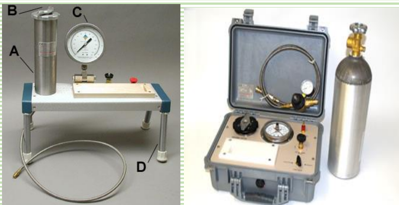
شکل ۸- نمونه هایی از دستگاه بمب فشاری
