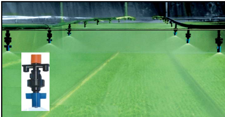
شکل ۱۰- ایجاد سرما با استفاده از سیستم مه پاشی
